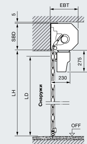
Диапазон размеров внутренних и внешних рулонных ворот
